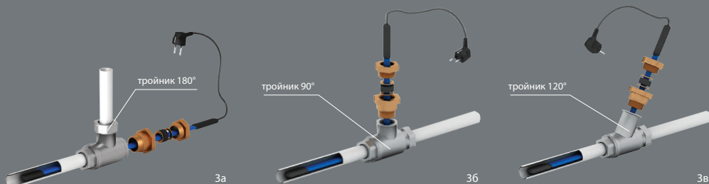
Рис.3. Схемы ввода нагревательной секции внутрь трубопровода: а - прямой ввод; б - ввод под углом 90°; в - ввод под углом 120°
