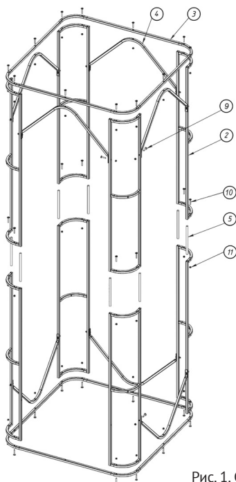
Рис. 1. Сборка каркаса.
